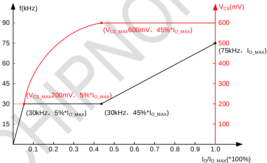
F_{OSC} 和 I_O 与负载的关系
