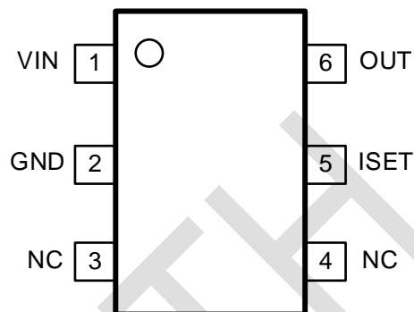
CN1502TER(SOT23-6)
