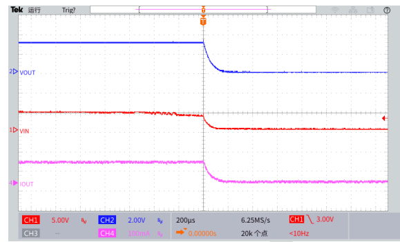
VIN 下电
