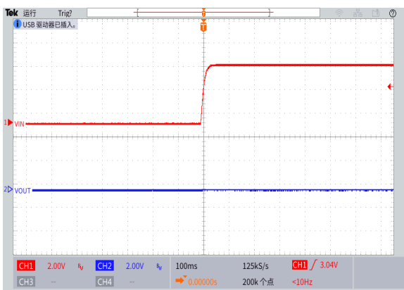
短路保护
