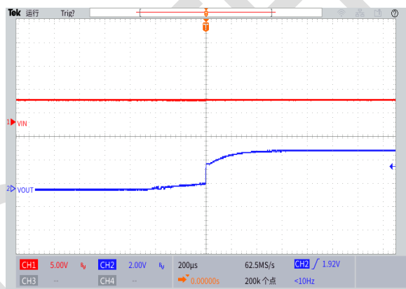
短路恢复
