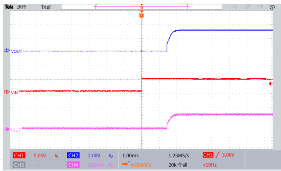
VIN 上电
