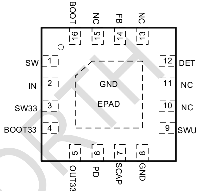
图 1 QFN4x4-16L
