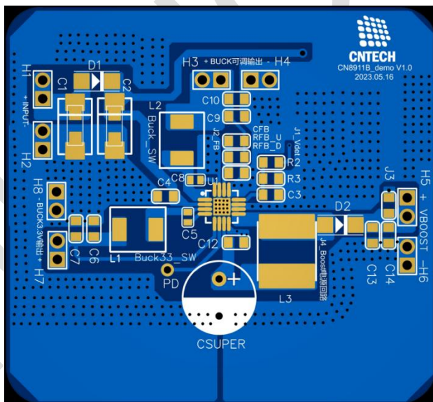
图 8 PCB 布局参考
